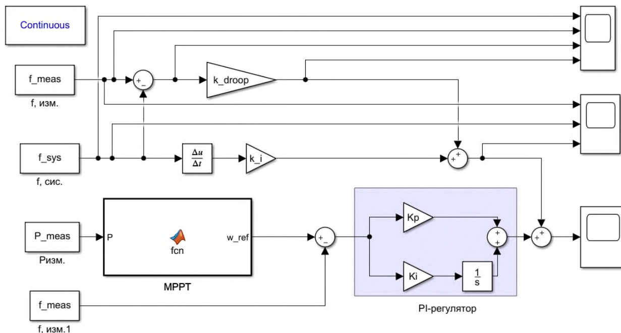
Рисунок 6 – Структурная модель управления инерцией от ВЭС
