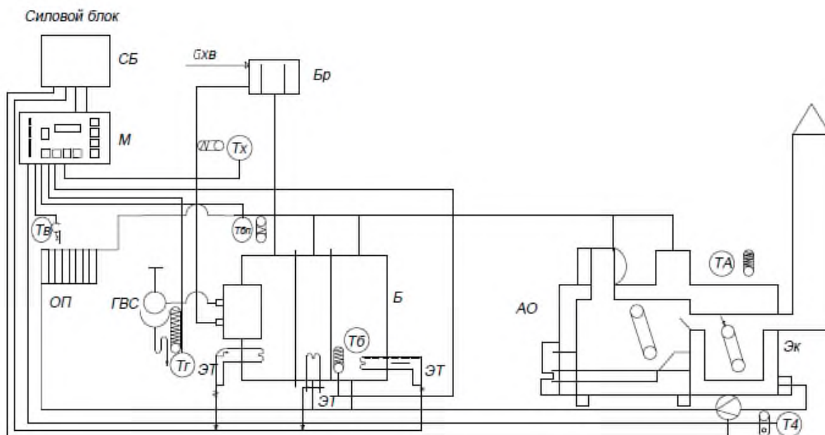
Расми 2 – Схемани гармидиҳии механикӣ: АО дастгоҳи гармидиҳӣ, ЭК-экомайзер; Б-бак аккумулятор бо электрокомпенсатори талафот; ГВС -таъминоти оби гарм; БР бак васеъкунанда; Гхв- таъмини оби хунук; М -микроконтроллер; СБ- блоки қувва; Т- табдилдиҳандаҳои аввалия
