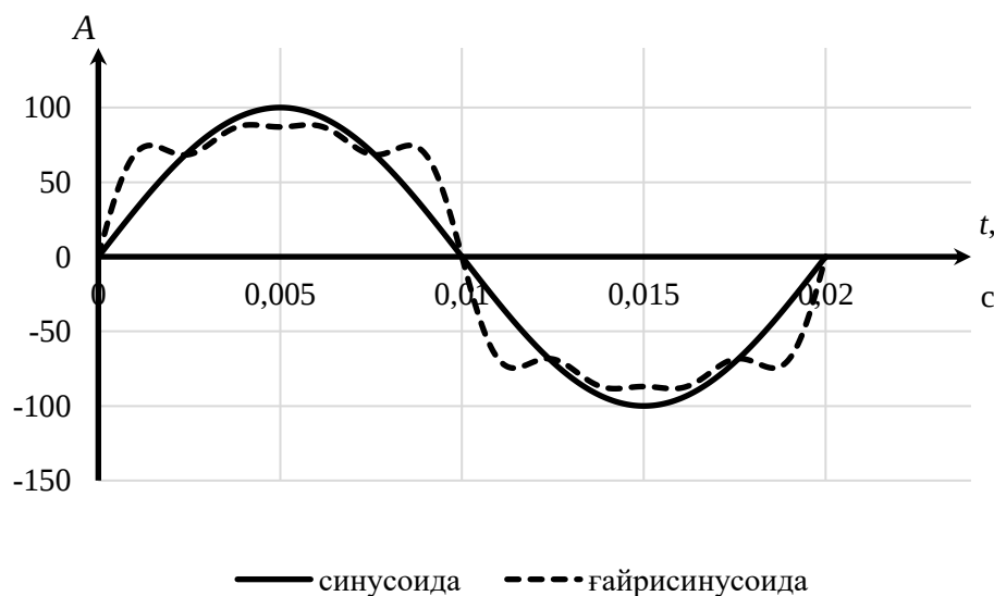
Расми 3 – Шакли қатъаттаи функсияи синусоидаӣ ва ғайрисинусоидаӣ
