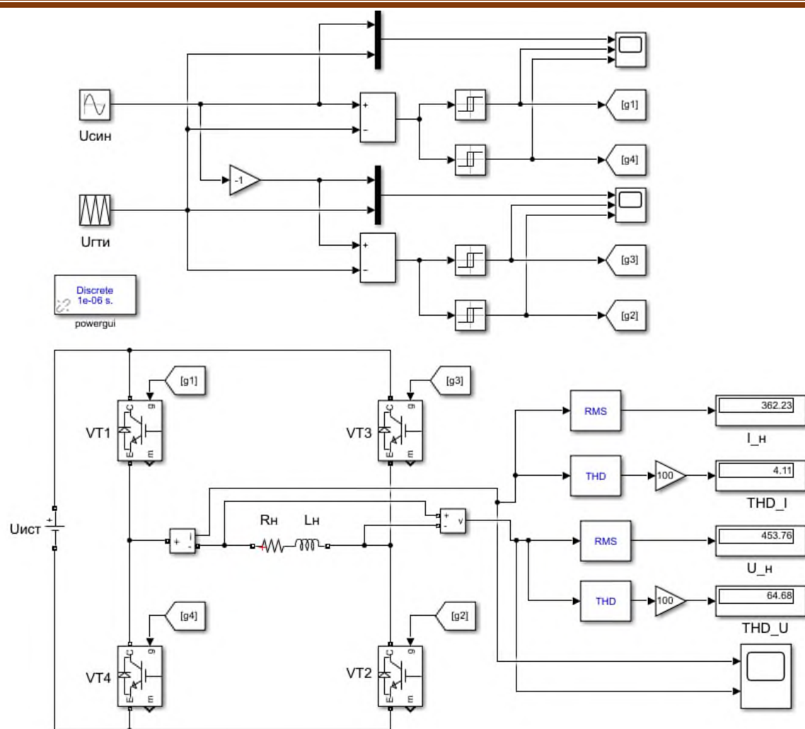
Рисунок 5 – Имитационная компьютерная модель унipoлярного инвертора с синусоидальной ШИМ
