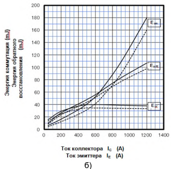
Рисунок 6 – Энергетические характеристики IGBT-транзистора типа CM600DX-24T1: а) ВАХ транзистора U_{ce}(I_c) ; б) зависимости энергии включения E_{on}(I_c) , выключения E_{off}(I_c) и восстановления обратного диода от тока эмиттера E_{rr}(I_e)
