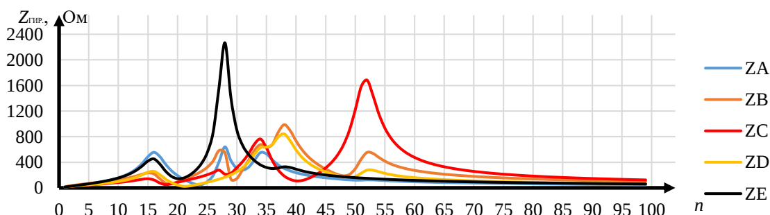
Расми 5 – Тавсифи амплитудавӣ-басомадии нақшаи озмоишӣ 5 – гиреҳи IEEE дар речаи муътадил (нормалӣ)
