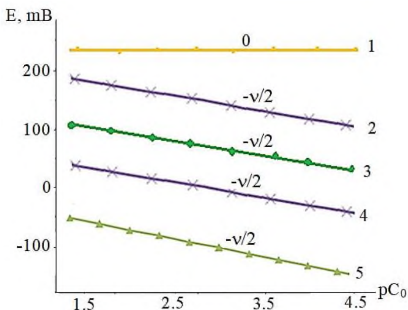
Рисунок 3 – Зависимость ЭДС (E, mV) системы Mn(II)–Mn(IV)–CH 3 COOH–C 2 H 5 OH от pC Mn(IV) при ионной силе раствора 1,0; C Mn(II) = 1·10 -4 и C HAc = 1·10 -3 моль/л; температуре 298,15 К. Кривые относятся к pH: 1 – 2,0; 2 – 3,5; 3 – 5,5; 4 – 7,0; 5 – 9,5.
