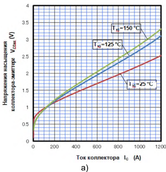
Рисунок 6 – Энергетические характеристики IGBT-транзистора типа CM600DX-24T1: а) ВАХ транзистора U_{ce}(I_c) ; б) зависимости энергии включения E_{on}(I_c) , выключения E_{off}(I_c) и восстановления обратного диода от тока эмиттера E_{rr}(I_e)
